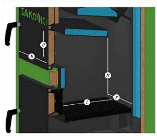
Рис.2 Размеры камеры сгорания котла SAKOVICH STANDART
