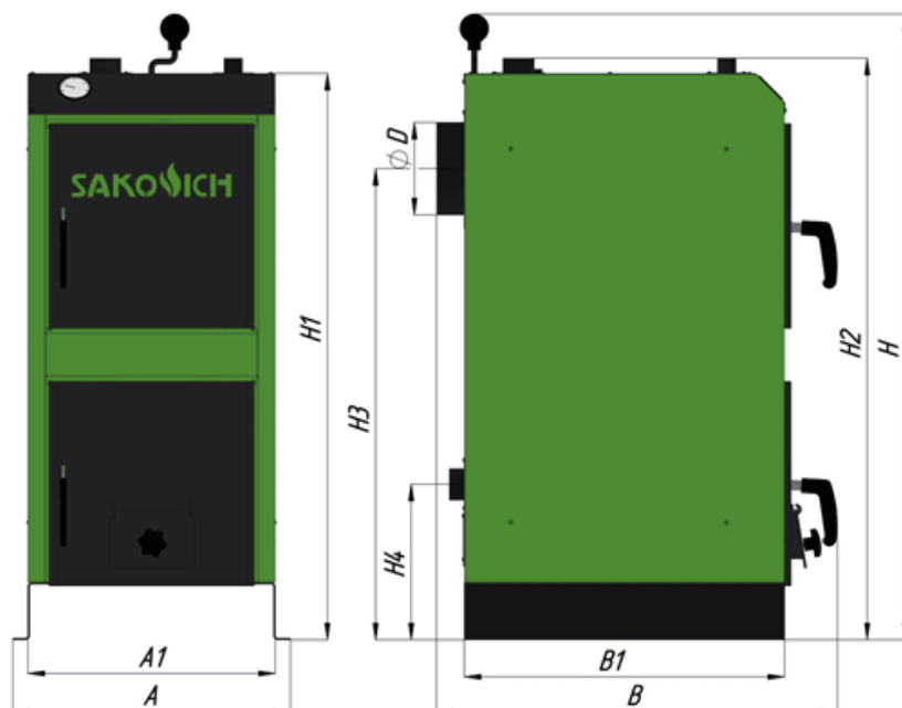
Рис.3 Размеры котла SAKOVICH STANDART
